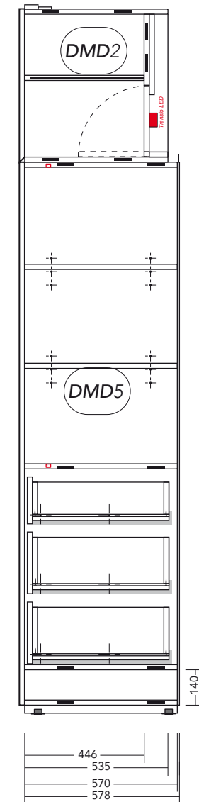
COUPE BB
