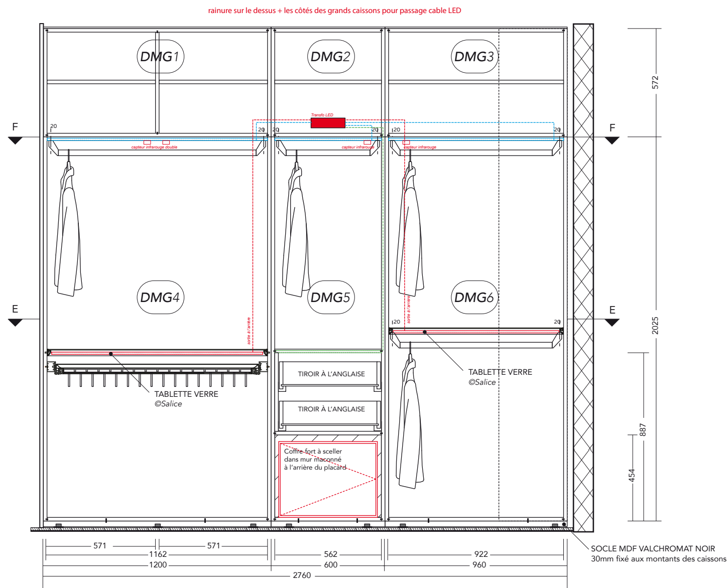
COUPE EE
