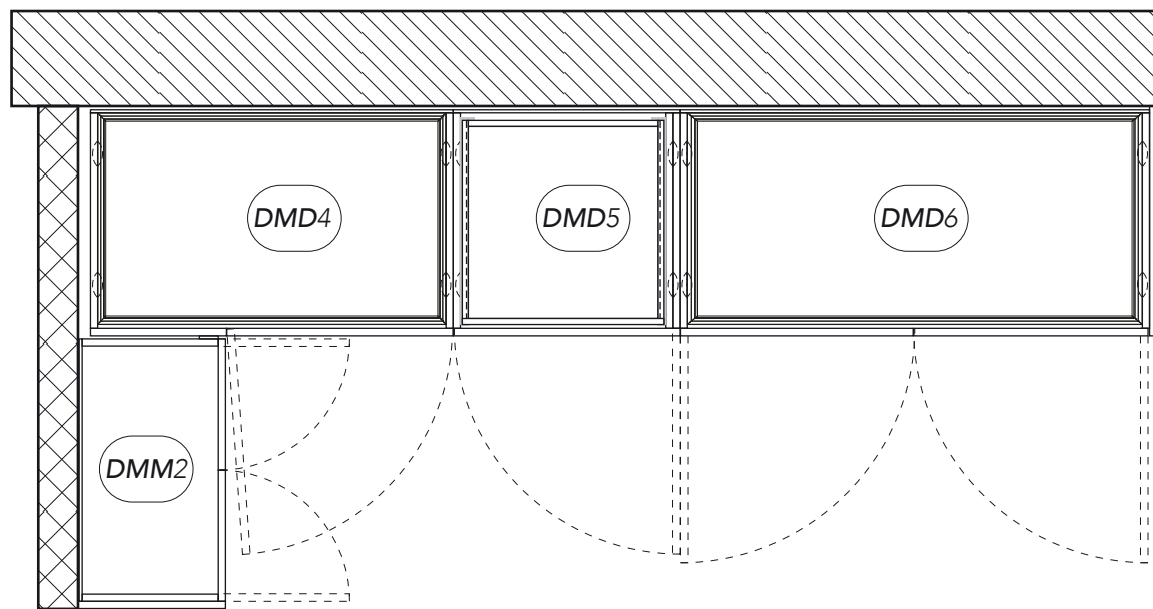
COUPE EE
