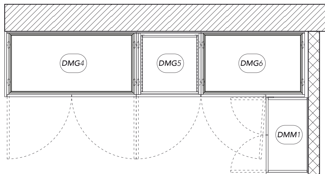
COUPE EE
