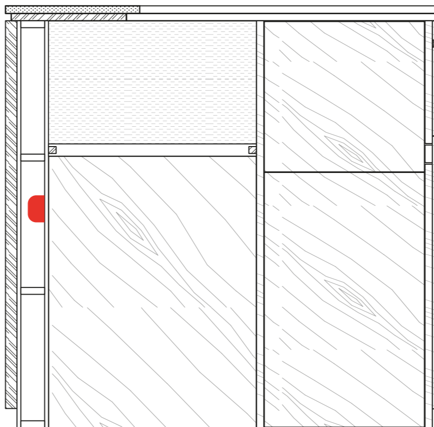
COUPE CC
